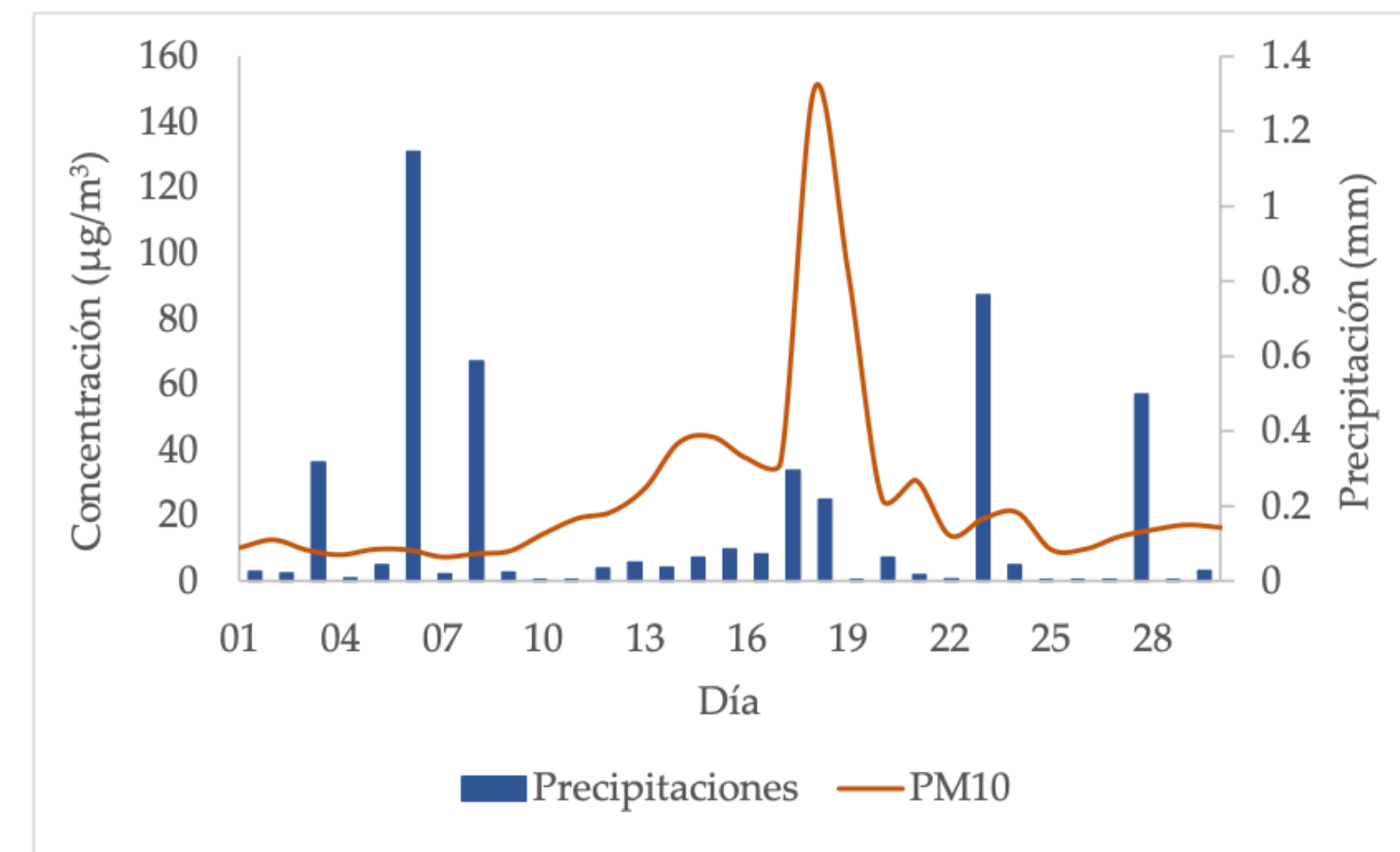
Imagen 11. Concentración de PM 10 y precipitación cada día del mes de julio de 2022.
